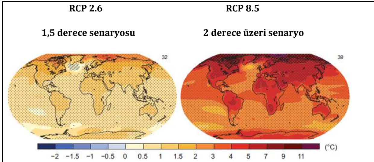
Şekil 1. 1986-2005 ve 2081-2100 Yılları Arasındaki Değişim
